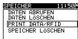
Bild 7.2: Speichermenü
