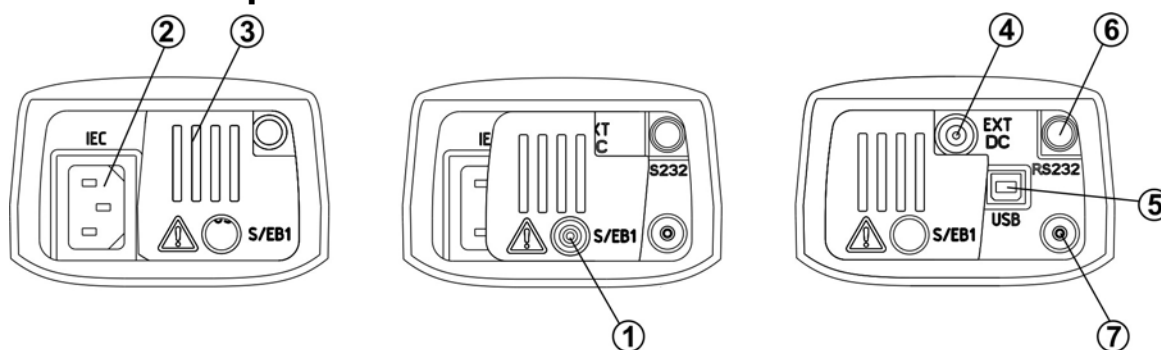
Bild 2.2: Anschlussplatte
